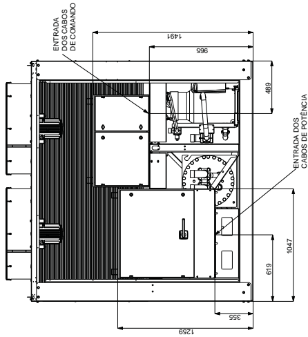
VISTA DO LADO DA CAIXA ELÉTRICA UNIDADES 30RSAT25 - 150 - 175 E 200
