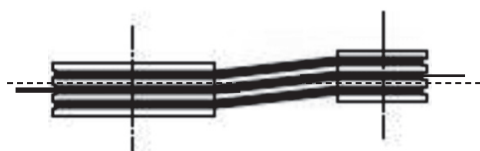
Fig. 21 - Alinhamento polia/correia
