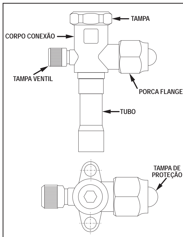
FIGURA 17 - VÁLVULA SERVIÇO LINHAS DE SUCÇÃO E EXPANSÃO
