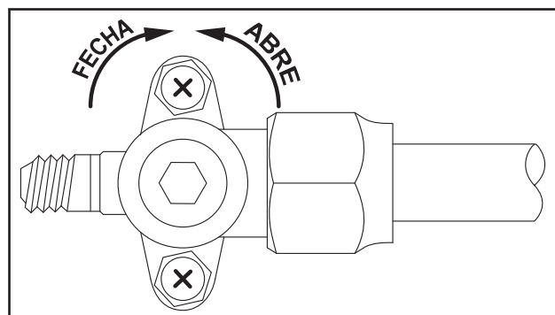
FIGURA 18 - VÁLVULA SERVIÇO SEM A PORCA DE PROTEÇÃO
