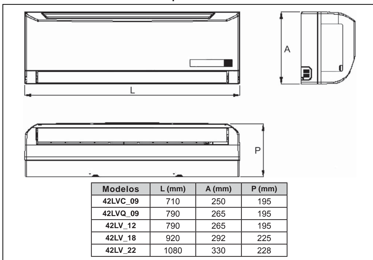
FIGURA 12 - DIMENSIONAL
